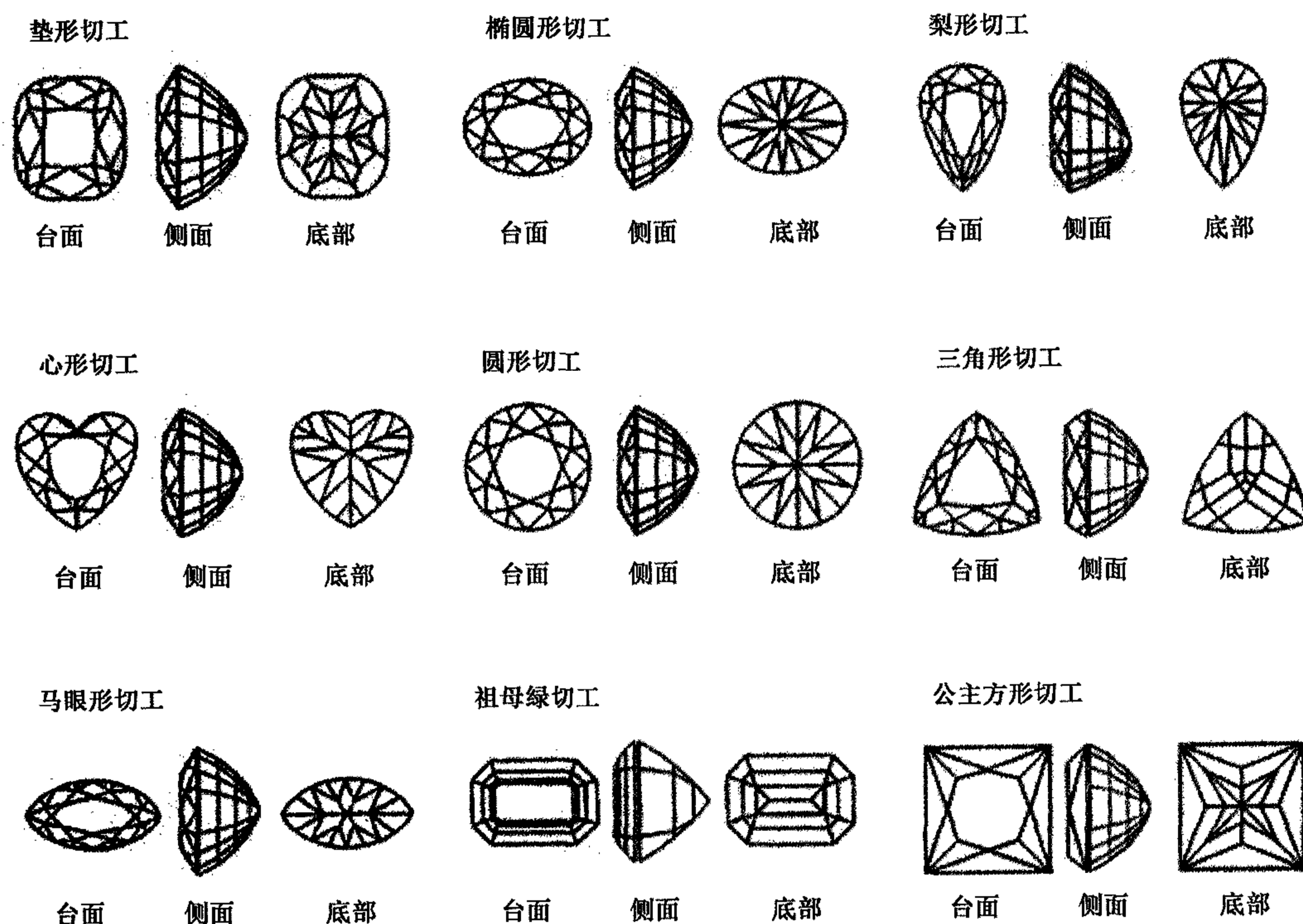
图 D.1 蓝宝石常见的切工类型
